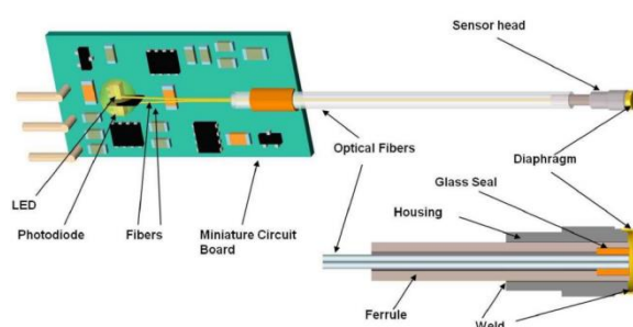
图1 传感器及信号调理器结构
