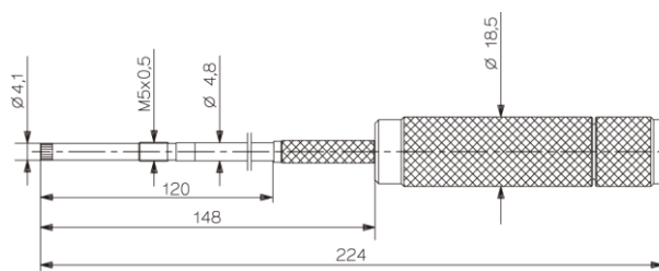
图8 密封面精整工具 1300A111
