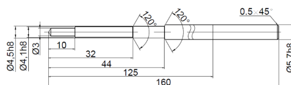
图7 台阶钻头 1300A18
