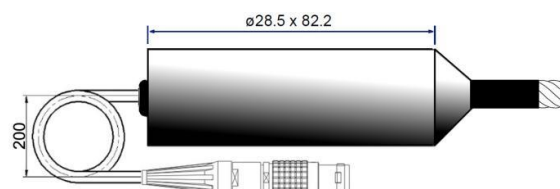
图5 信号调理器
