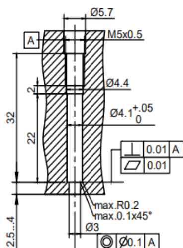
图3 OP058A 传感器安装孔
