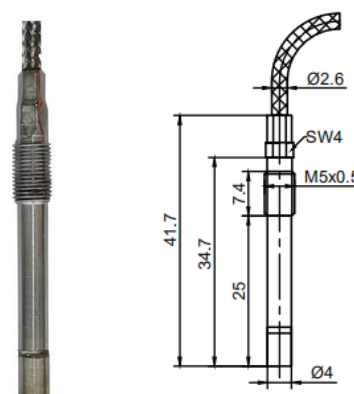
图2 传感器外形及尺寸
